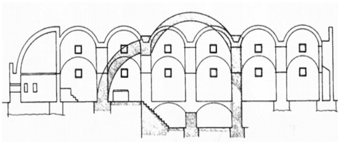
Rilievo della basilica di San Leucio
