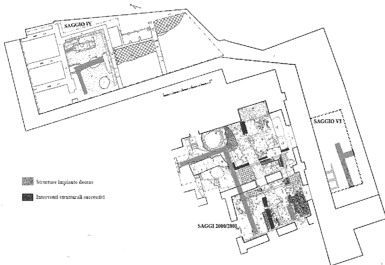
Fig. 11. Planimetria generale ricostruttiva con ubicazione delle strutture relative alla fase d'impianto della domus e degli interventi edilizi che si sono succeduti. Elaborazione grafica di P.Palazzo.
