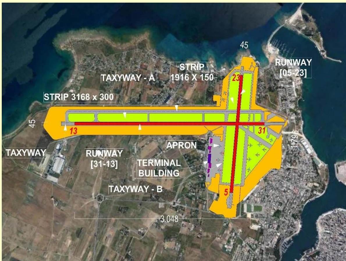
L'Aeroporto di Brindisi con le sue due piste incidenti, una da sudovest a nordovest e l'altra da nordest a sudest
